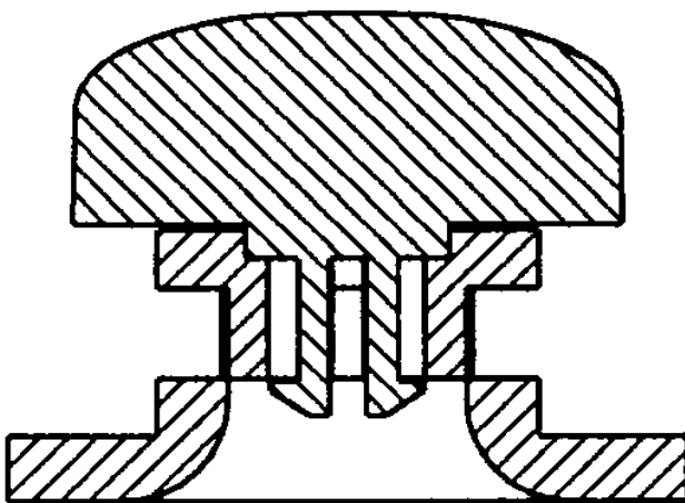
【F-F' 線拡大断面図】
