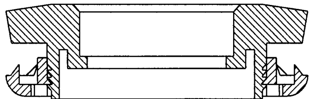
【G-G' 線拡大断面図】
