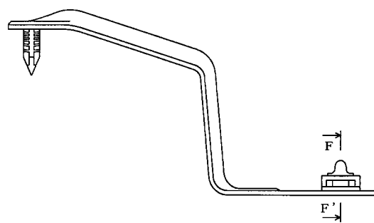
【雄部正面図】
