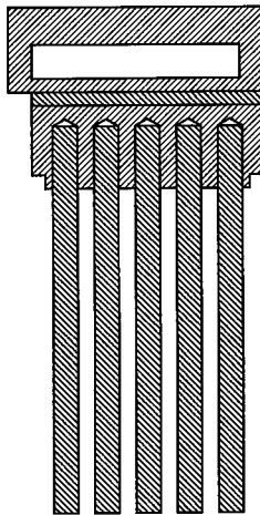
【C-C線断面図】
