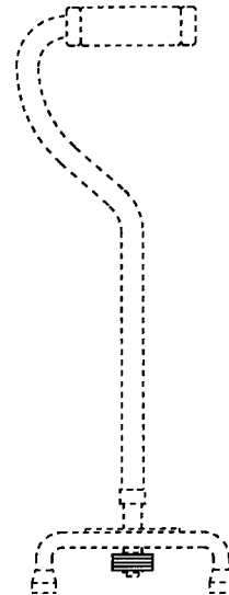
【左側面図】
