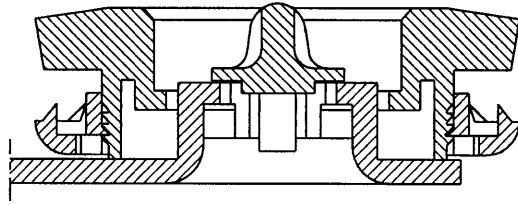
【A-A' 部分 B-B' 線拡大断面図】
