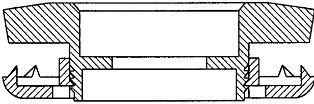
【H－H'線拡大断面図】
