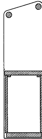
【B-B' 線断面図】
