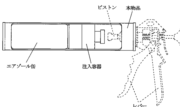
【使用状態を示す参考正面図】
