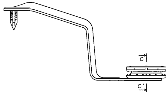
【正面図】
