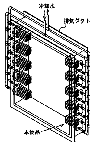
【使用状態を示す参考斜視図】
