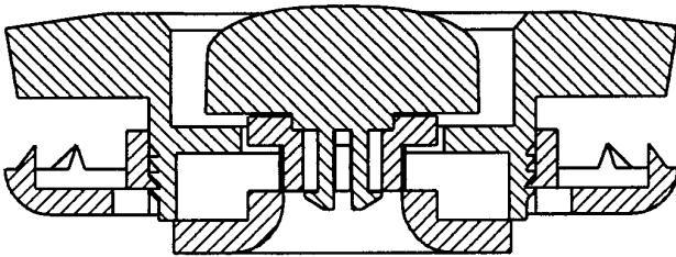
【C-C' 線拡大断面図】
